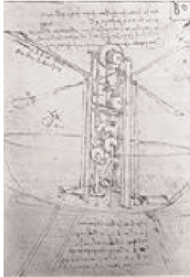
دیزاینیک بۇ (مەكىنەى فرين)، ۱۴۸۷، ۱۷، ۶x۲۳، ۵ سم، كاغەز، پەيمانگەى فرەنساىى. (ليۇناردو داڧنشى)
